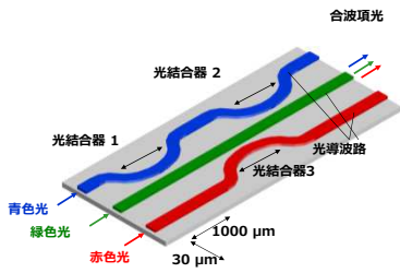
光導波路型合波器の構造
